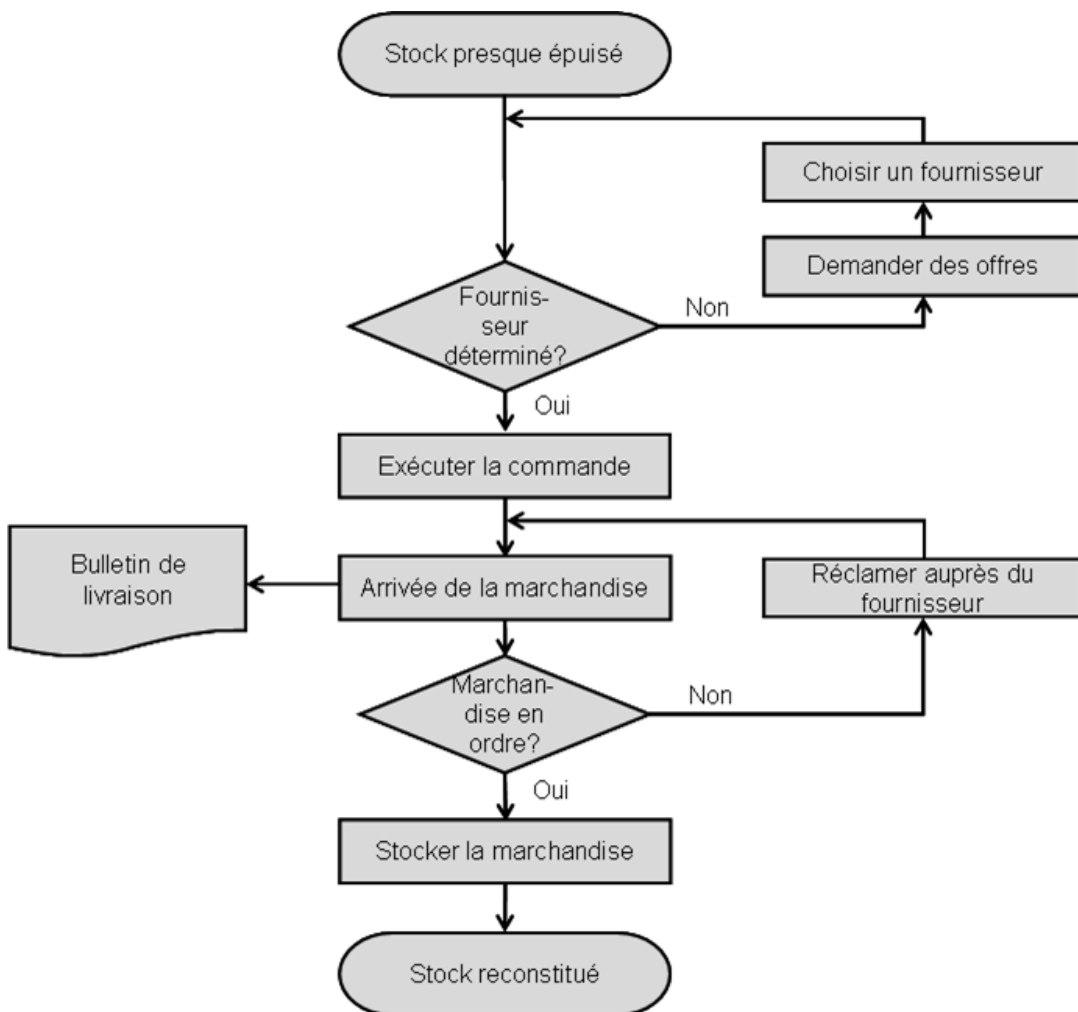
Illustration3:Exemple d'ordinogramme
